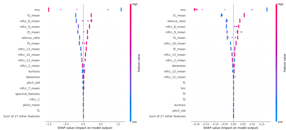
(a) Agrupación de las gráficas SHAP del clasificador.
