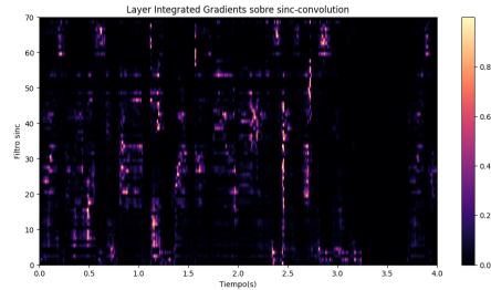
(b) Mapa filtro-tiempo normalizado generado con IG.
