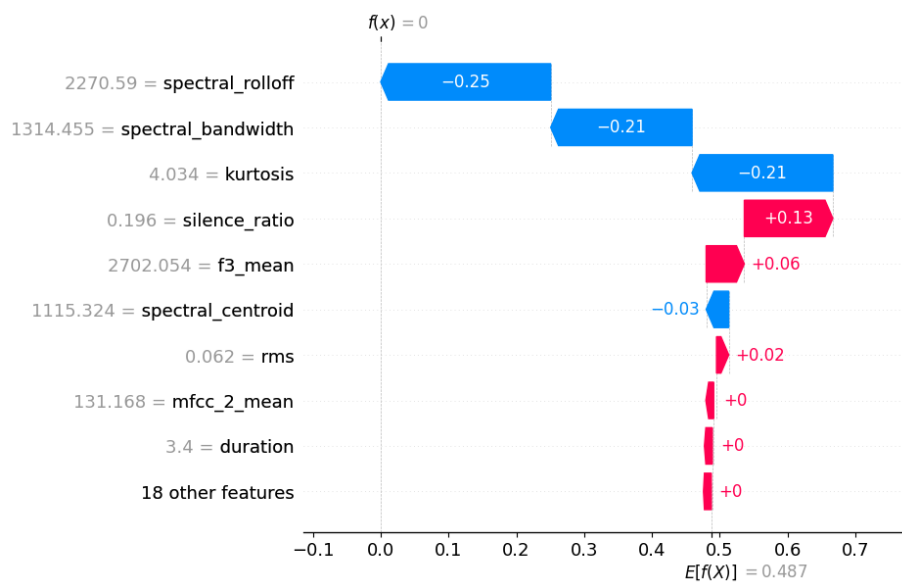
Figura 61: Explicación local con SHAP tras quitar spectral flatness y mfcc 1
