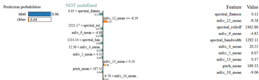
Figura 69: Explicación local con LIME
