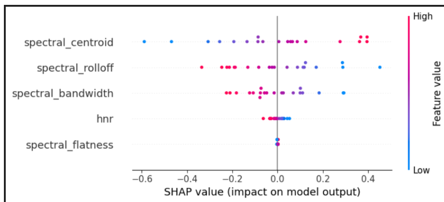
Figura 24: Shap global espectrales.
