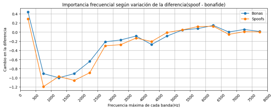
Figura 16: Resultados de margen de la ocultación frecuencial en AASIST.
