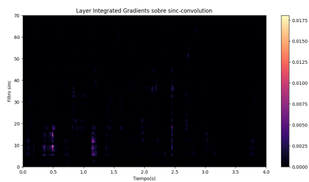
(a) Mapa filtro-tiempo generado con IG.
