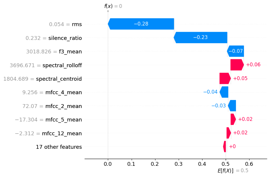
Figura 54: Explicación local con SHAP tras quitar spectral flatness, mfcc 1 y spectral bandwidth
