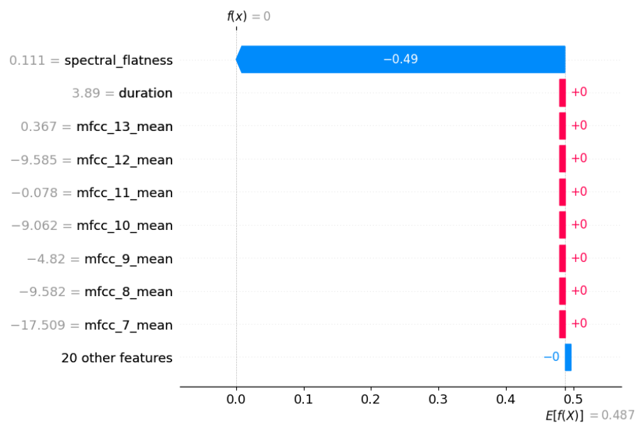
Figura 56: Explicación local con SHAP
