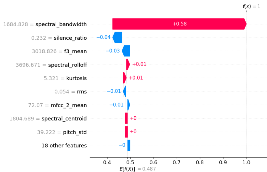
Figura 60: Explicación local con SHAP tras quitar spectral flatness y mfcc 1
