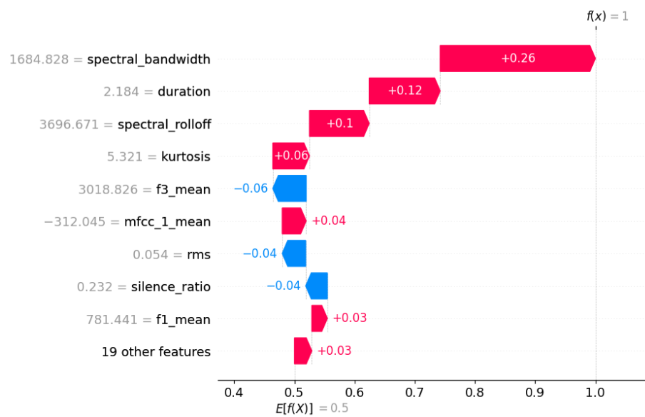
Figura 52: Explicación local con SHAP tras quitar spectral flatness
