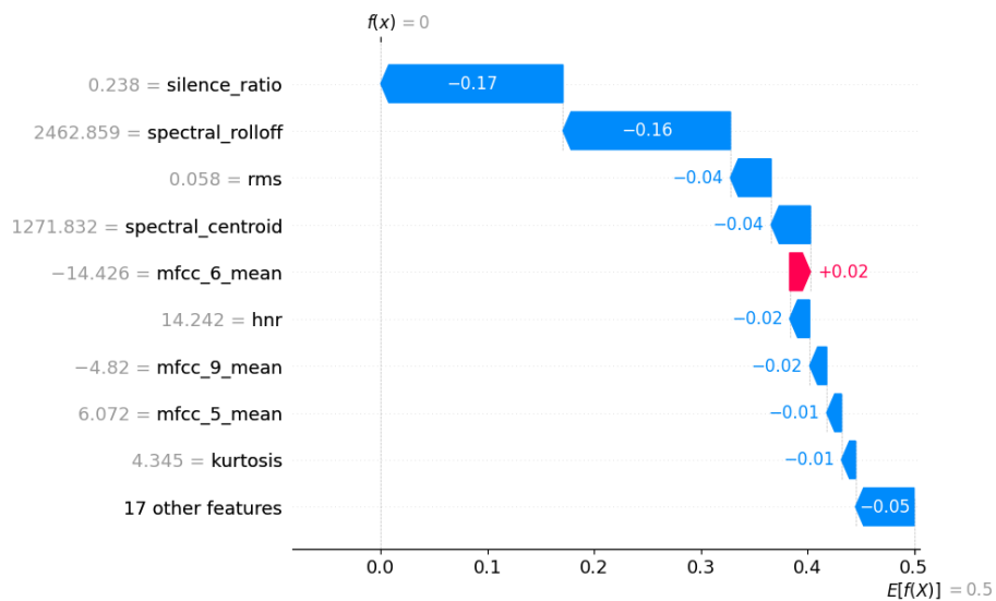
Figura 53: Explicación local con SHAP tras quitar spectral flatness, mfcc 1 y spectral bandwidth
