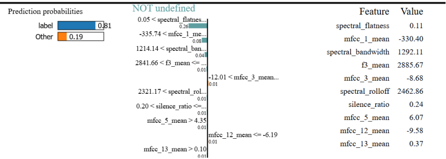
Figura 62: Explicación local con LIME
