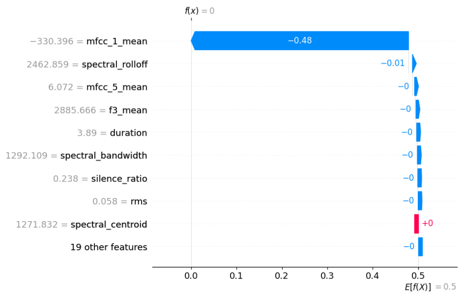
Figura 58: Explicación local con SHAP tras quitar spectral flatness
