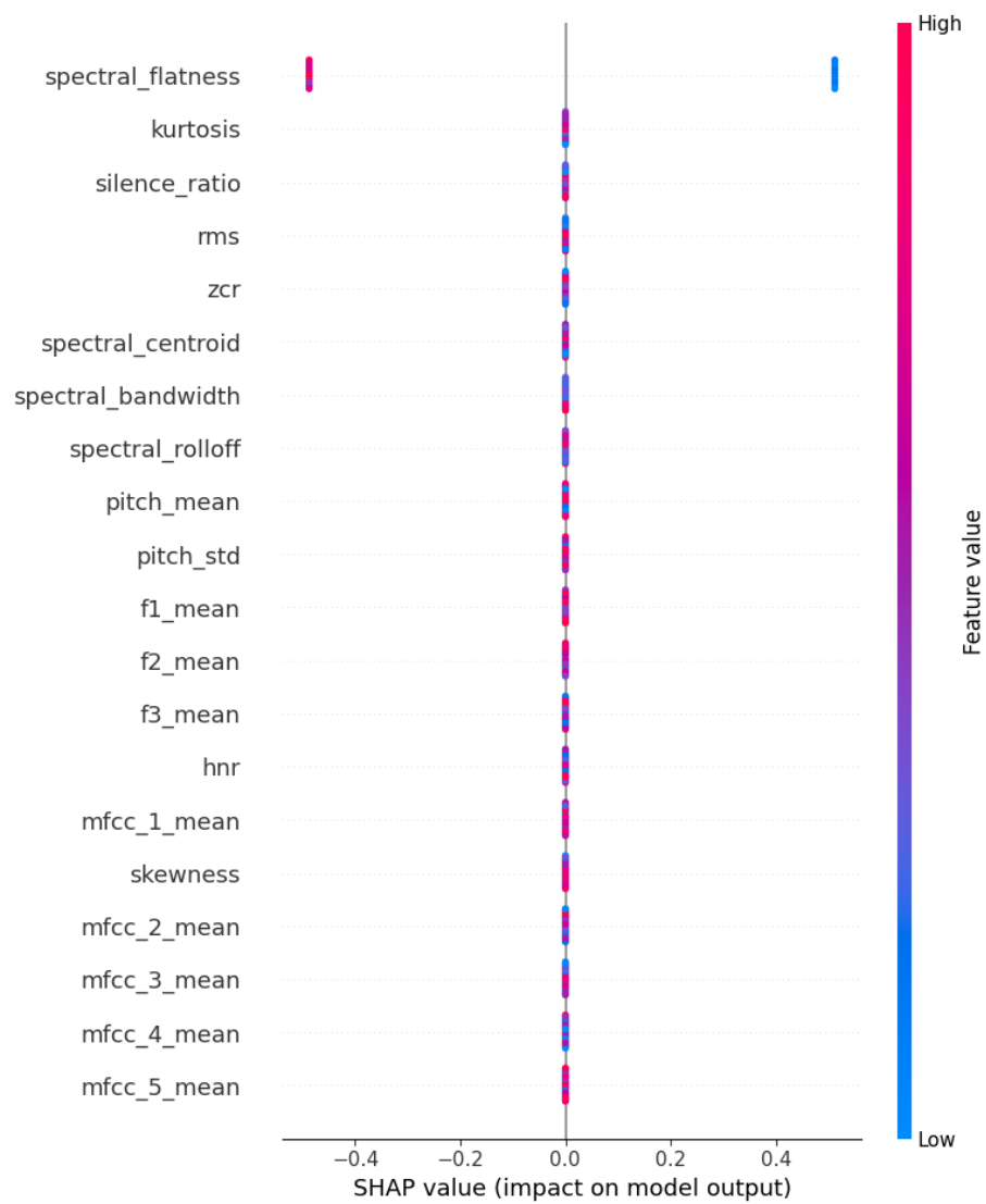
Figura 57: Explicación global con SHAP
