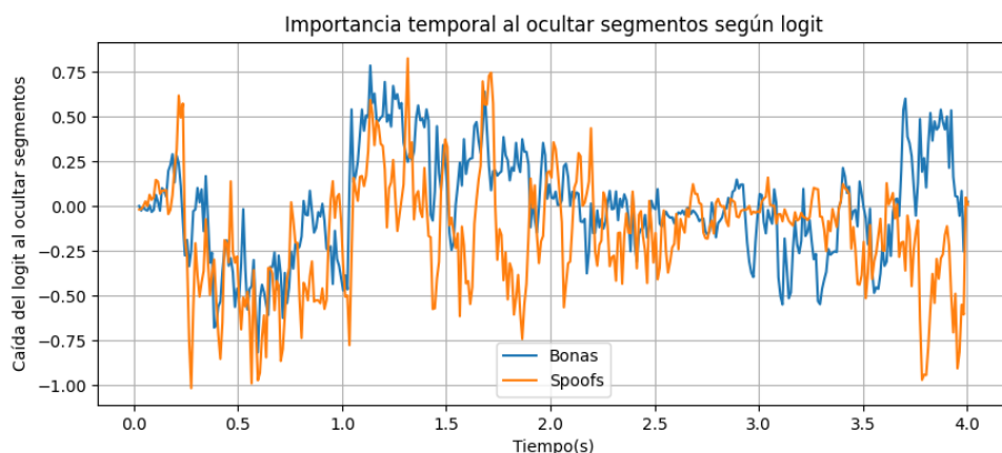
Figura 13: Resultados de “logit” de la ocultación temporal en AASIST.
