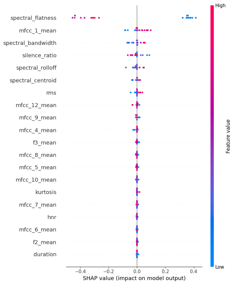
Figura 50: Explicación global con SHAP
