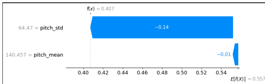
Figura 27: Ejemplo concreto (I_12_N).
