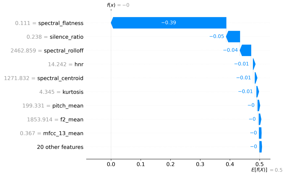
Figura 49: Explicación local con SHAP
