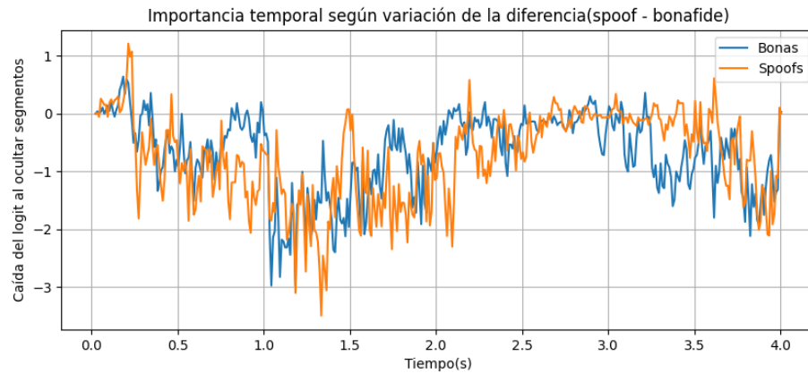
Figura 14: Resultados de margen de la ocultación temporal en AASIST.
