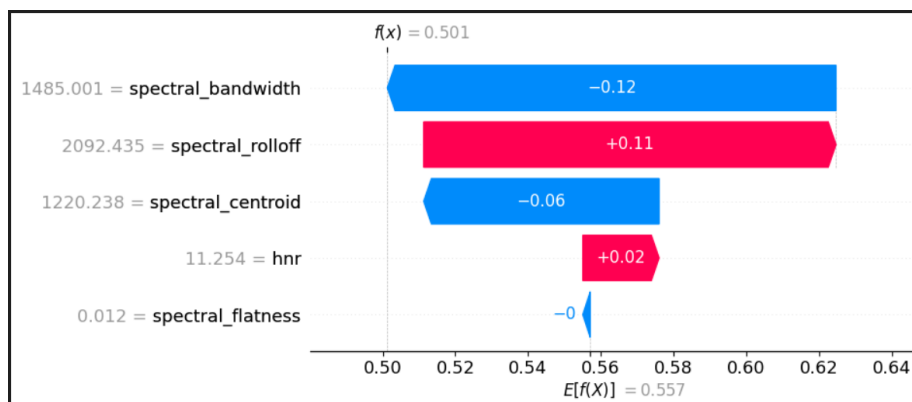
Figura 25: Ejemplo concreto (I_12_N).
