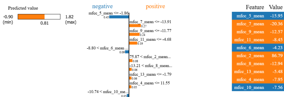
Figura 36: Explicación local mfccs Lime.
