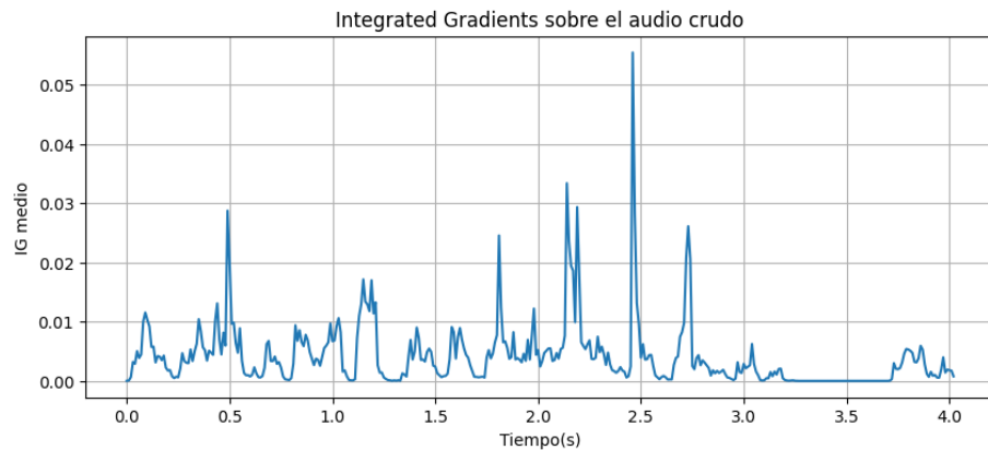
Figura 11: Importancia temporal al aplicar IG sobre audio.
