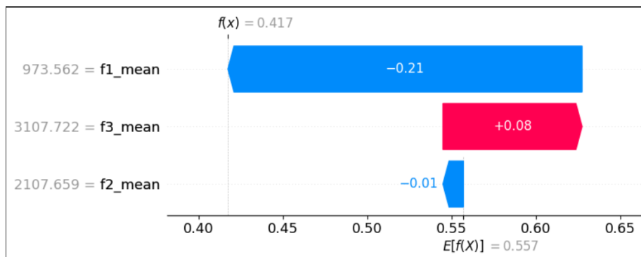
Figura 29: Ejemplo concreto (I_12_N).
