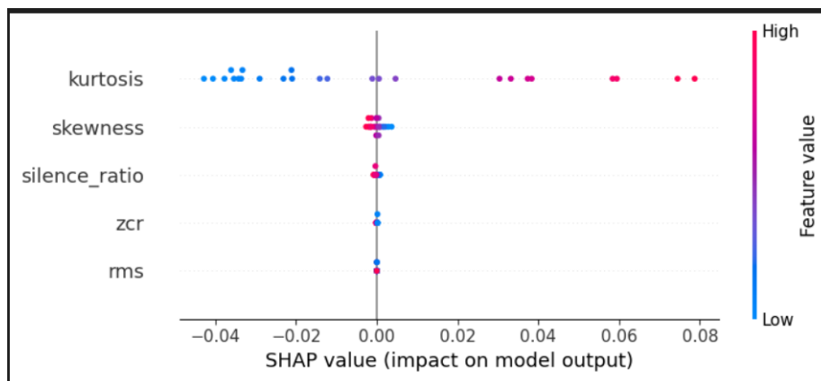
Figura 22: Shap global energía.
