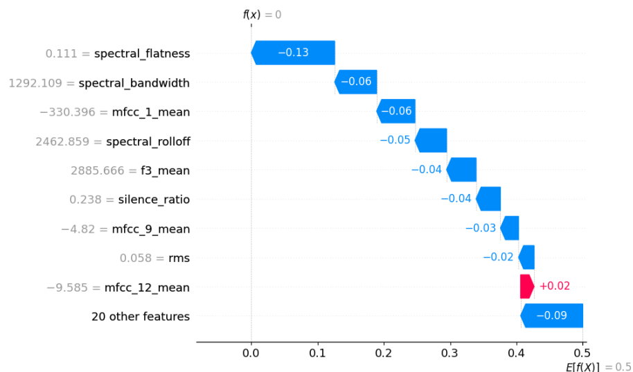
Figura 63: Explicación local con SHAP
