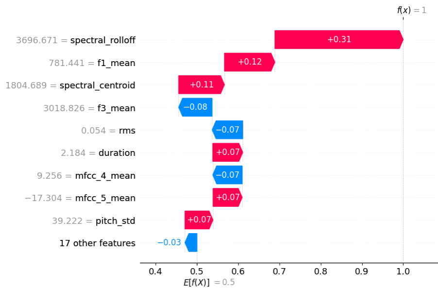
Figura 68: Explicación local con SHAP tras quitar spectral flatness, mfcc 1 y spectral bandwidth
