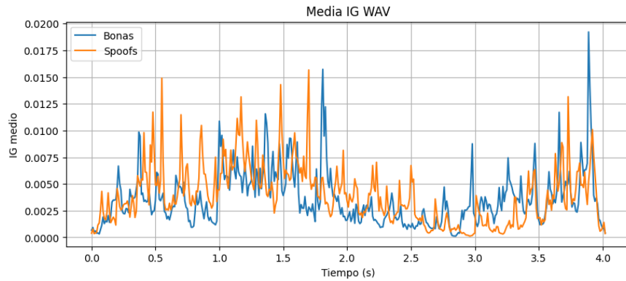
Figura 20: Importancia temporal al aplicar IG sobre audio.
