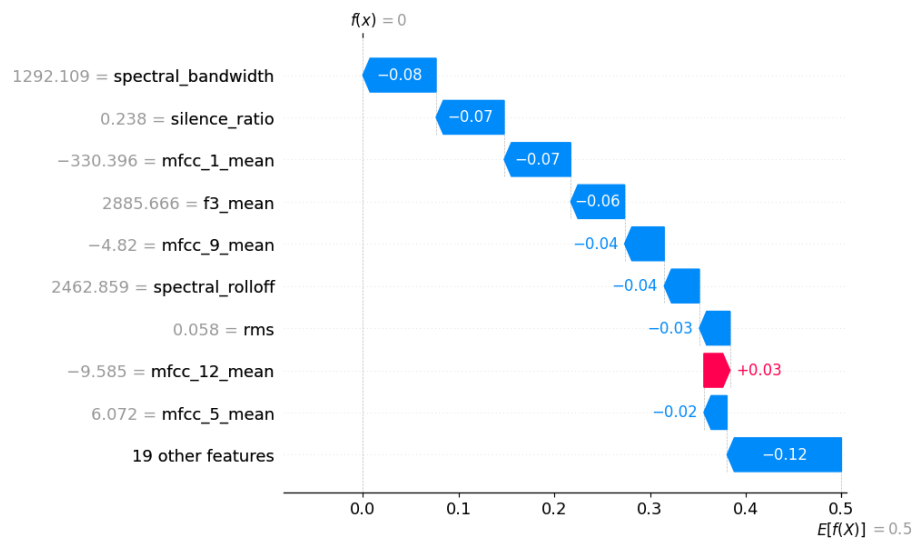
Figura 65: Explicación local con SHAP tras quitar spectral flatness
